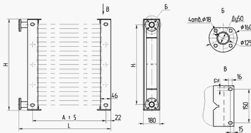
Рисунок 7. Габаритно-присоединительные размеры ТБЗ- ...
