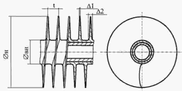
Рисунок 20. Биметаллические ТОЭ.
