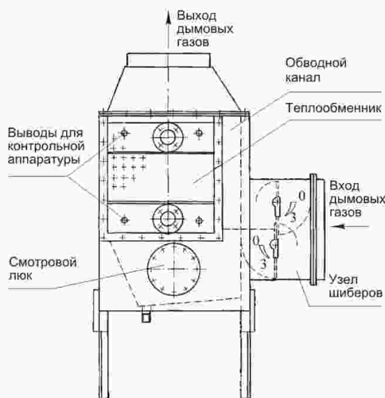
Рисунок 18. Эскиз общего вида газового конденсора
