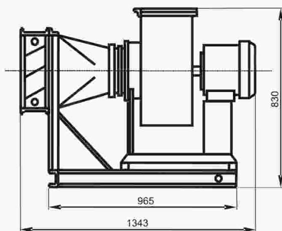
Рисунок 18. Габаритные размеры установок ВУ
