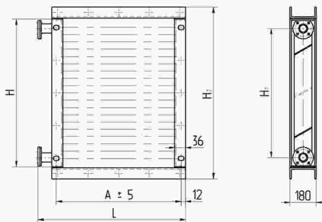
Рисунок 8. Габаритно-присоединительные размеры ВНВ113 ...
