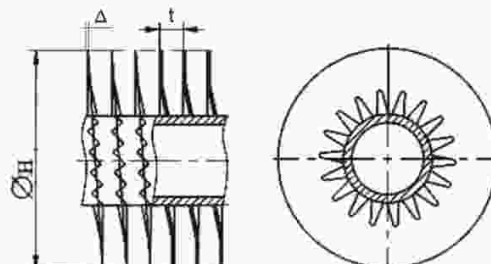
Рисунок 23. ТОЭ с навивным оребрением из стальной ленты
