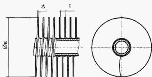
Рисунок 22. ТОЭ с навивным оребрением из алюминиевой или медной ленты
