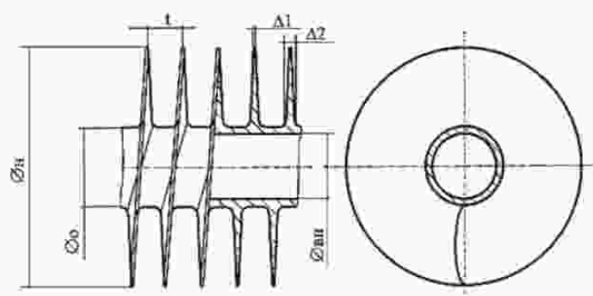
Рисунок 21. Монометаллические ТОЭ.
