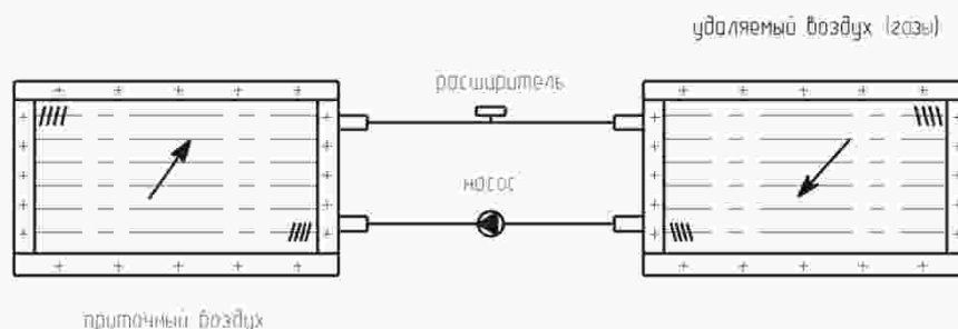
Рисунок 1. Схема применения калориферов в качестве теплоутилизаторов
