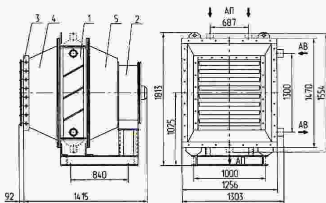
Рисунок 10. Агрегаты АВ(П)-21-... 1 – воздухонагреватель; 2 – осевой вентилятор; 3 – жалюзи; 4 – конфузор; 5 – диффузор.
