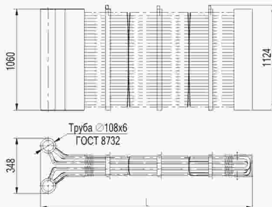
Рисунок 6. Габаритные размеры секций СО
