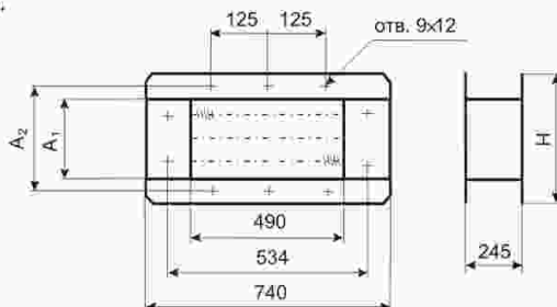
Рисунок 11. Габаритно-присоединительные размеры ВЭ
