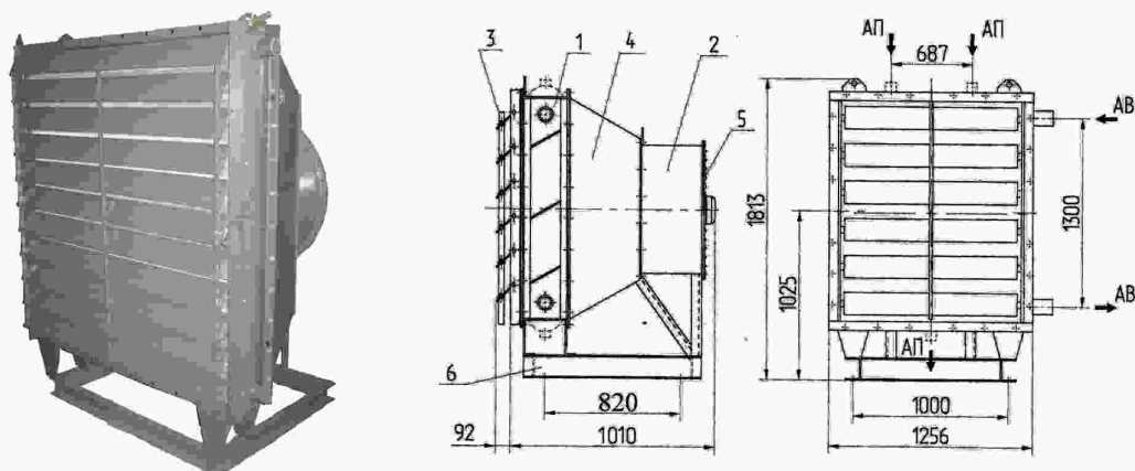
Рисунок 10. Агрегаты АВ(П)-25-...
